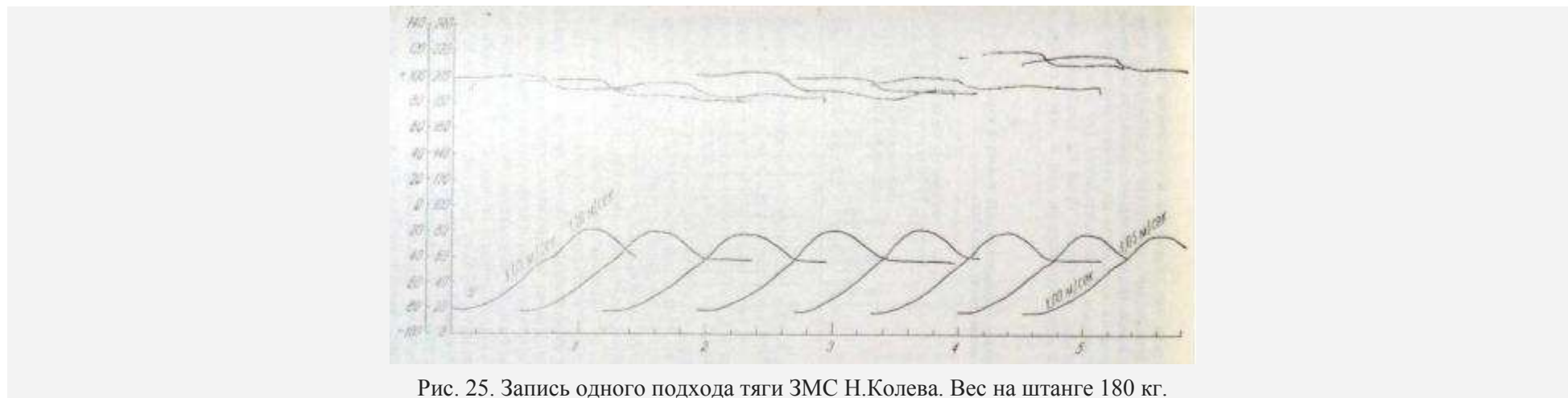
Рис. 25. Запись одного подхода тяги ЗМС Н.Колева. Вес на штанге 180 кг.
